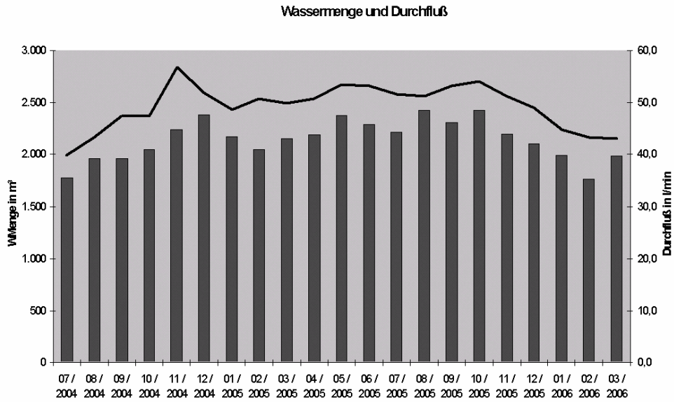
Abb. 10: Wassermenge und Durchfluß.
