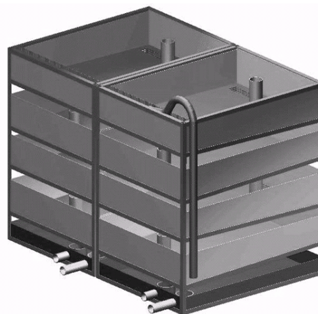
Abb. 4: Wannensstapel.
