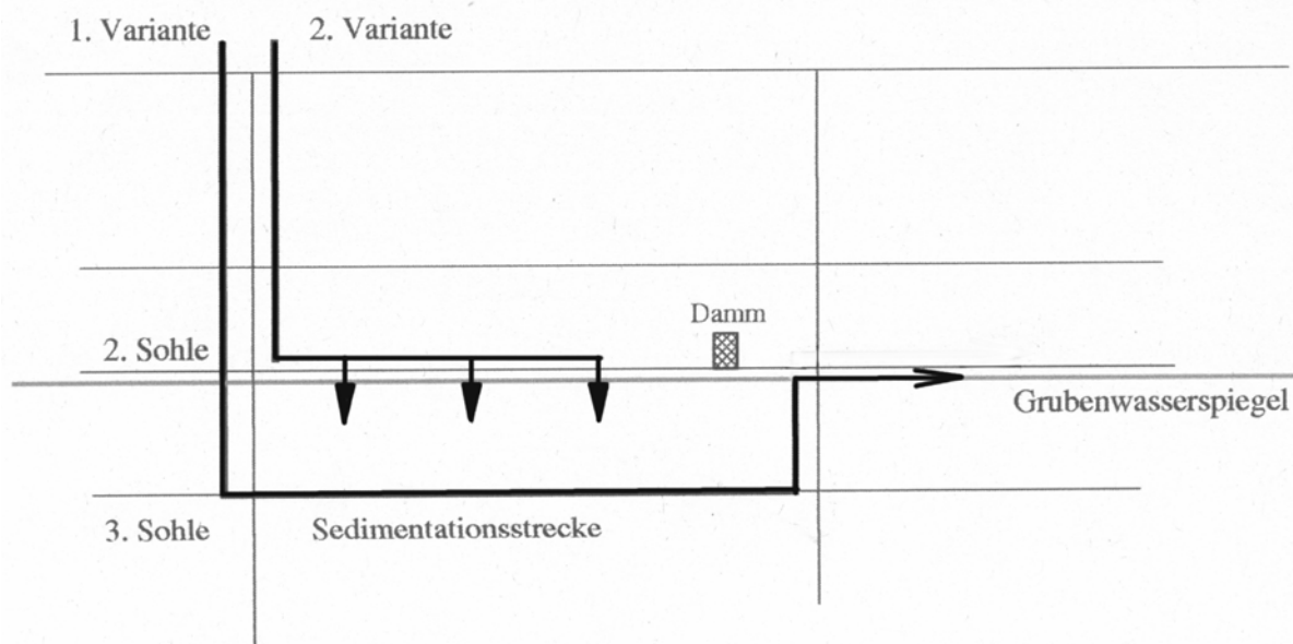
Abb. 2: Versuchskonzepte für den Versturz von Haldensickerwässern in den gefluteten Grubenraum.
