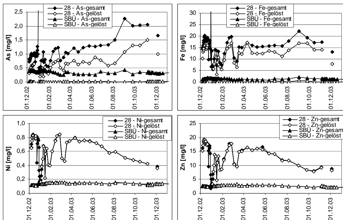
Abb. 5: Zeitliche Entwicklung der As-, Fe-, Ni- und Zn-Konzentrationen am Versturzpunkt (28) und am Gesenk 2. Sohle (SBU).
